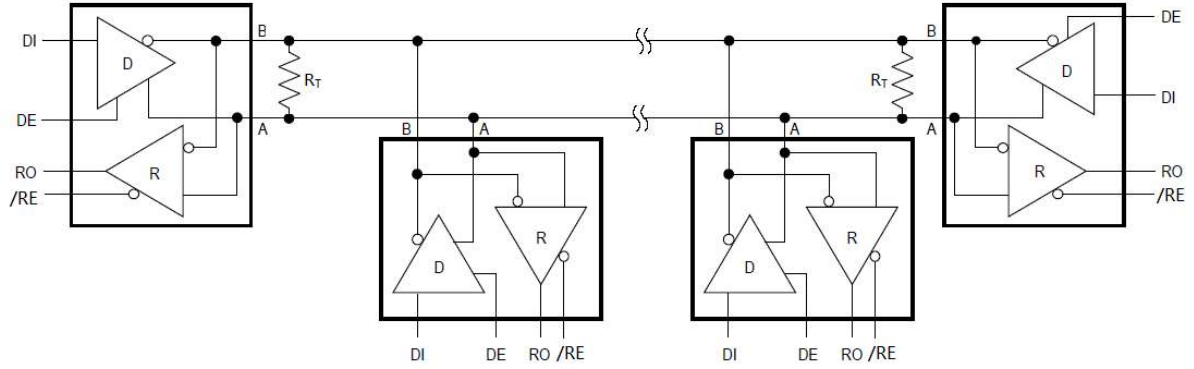
图10 典型半双工RS-485网络
